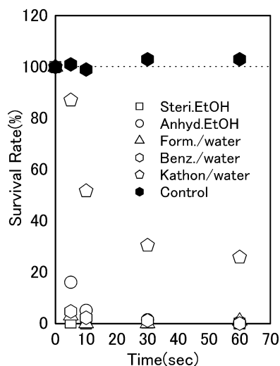
図1 各薬剤の真菌への殺菌消毒効果
