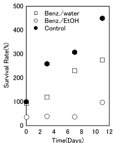
図7 塩化ベンザルコニウムによる石材試験体への殺菌効果
