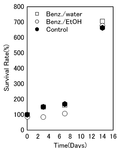
図6 塩化ベンザルコニウムによる土壌試験体への殺菌効果
