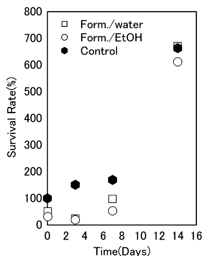
図4 ホルマリンによる土壌試験体への殺菌効果
