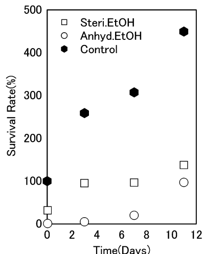
図3 エタノールによる石材試験体への殺菌効果
